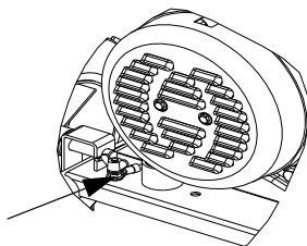
Figure 3-1. La mise à la terre de la génératrice
