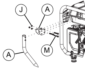
Figura 2-11. Conjunto de manilla
