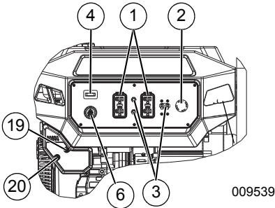
Figura 2-3. Panel de control de PM9400E con arranque eléctrico
