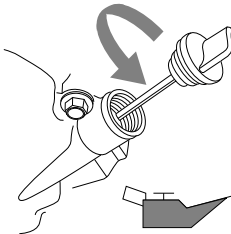
Figure 2-14. Sortir la jauge à huile
