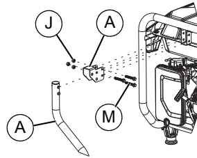
Figure 2-11. Assemblage de la poignée
