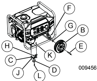
Figura 2-10. Conjunto de pata y rueda
