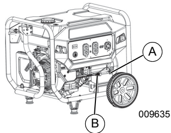
Figure 4-6. Raccordement des câbles de batterie
