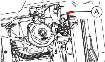
Figure 3-4. Levier du volet de départ
