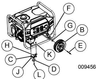
Figure 2-10. Assemblage des roues et des pieds
