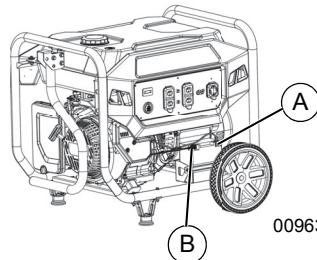
Figura 2-12. Conexión de los cables de la batería
